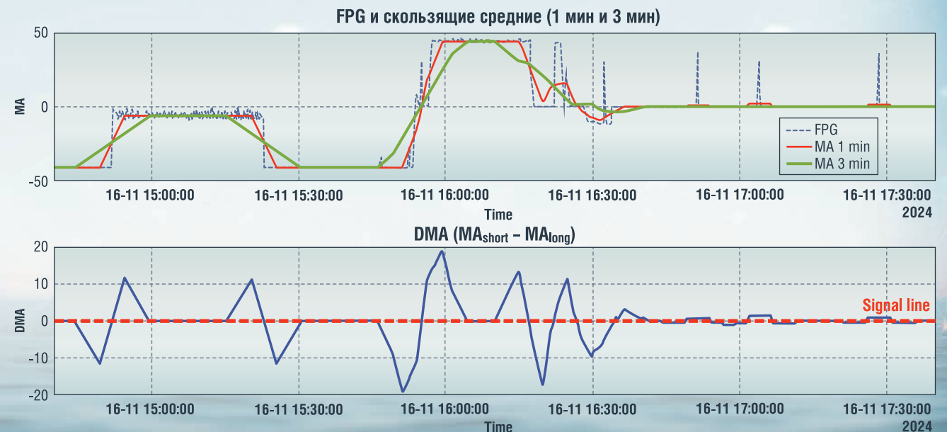
РИСУНОК 3. Реакция FPG и скользящих средних с различными временными интервалами. В нижней части графика отображена производная характеристика (DMA), позволяющая оценить краткосрочную динамику в контексте долгосрочного тренда
