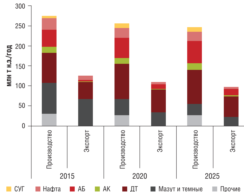
РИС. 5. Прогноз производственного и экспортного потенциала нефтеперерабатывающей отрасли России
